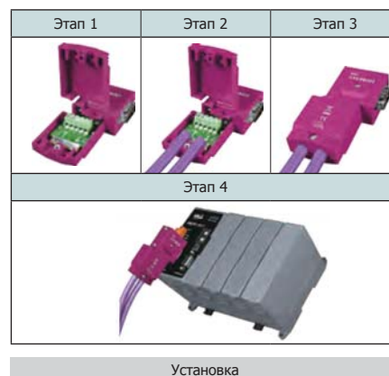
Опционально: PROFIBUS разъем: CNT-PROFI
