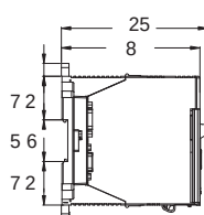
Вид слева
